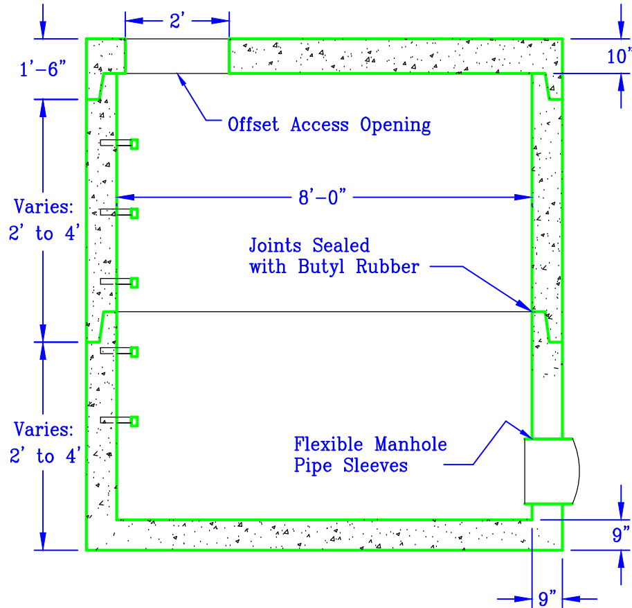
SECTION A-A
