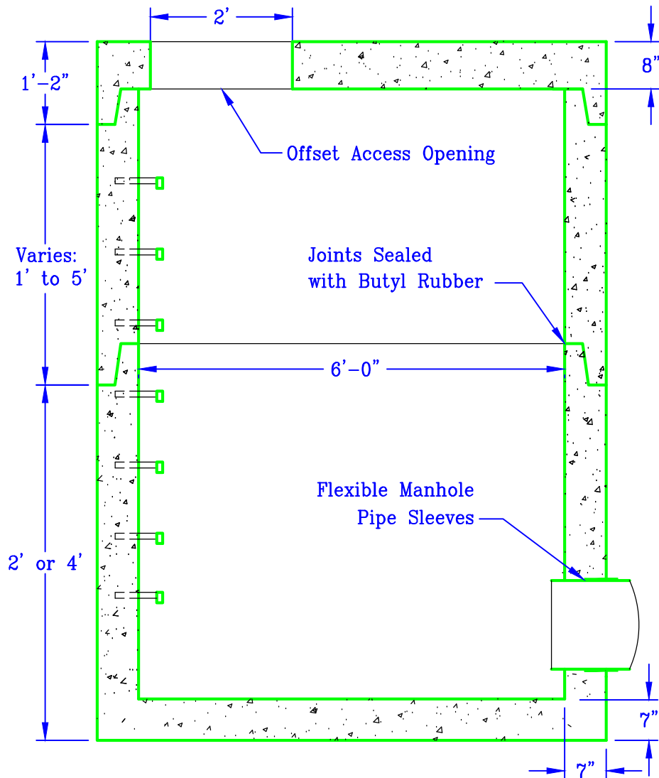
SECTION A-A
