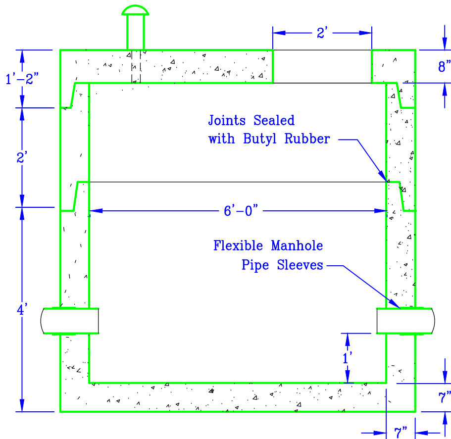
SECTION A-A
