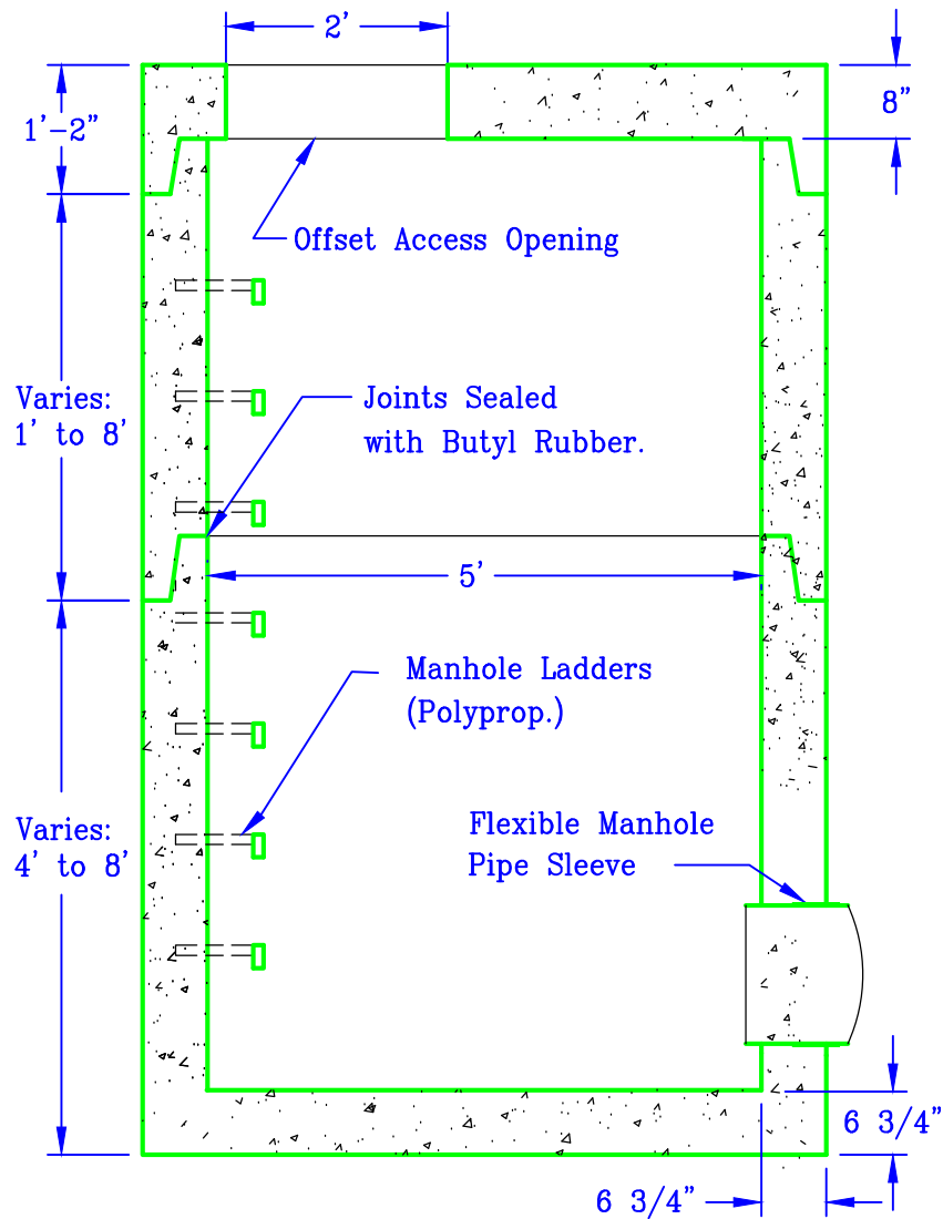
SECTION A-A
